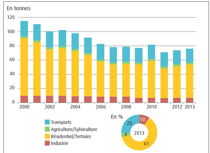
Graphique 23 : évolution des émissions françaises de HAP
