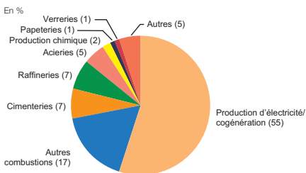
Répartition des émissions par secteur en 2013 (total : 1 925 Mt CO 2 )
