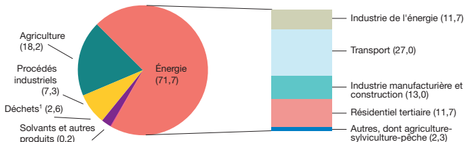
Répartition par source des émissions de GES en France en 2012 (DOM inclus) (490 Mt CO 2 éq. hors UTCF 2 )
